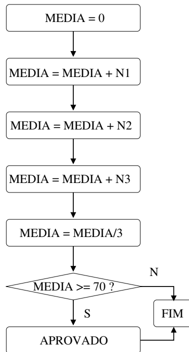
Figura 1: Fluxograma preliminar para cálculo da média das notas.
