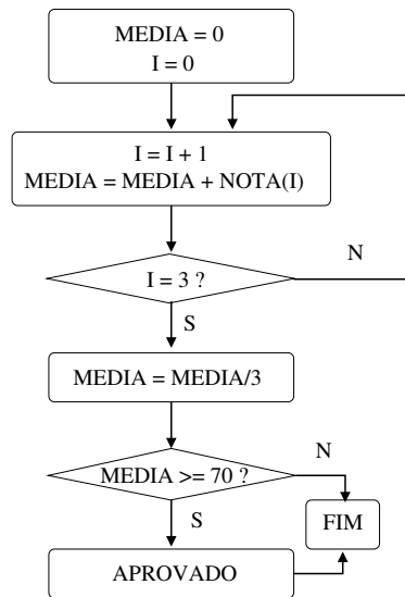
Figura 2: Fluxograma atualizado para cálculo da média das notas.
